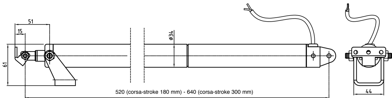
Actuators dimensions
